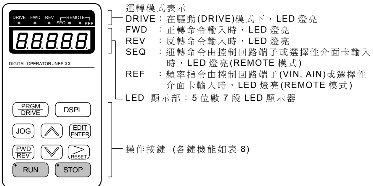
圖 10 LED 操作器各部名稱及機能
