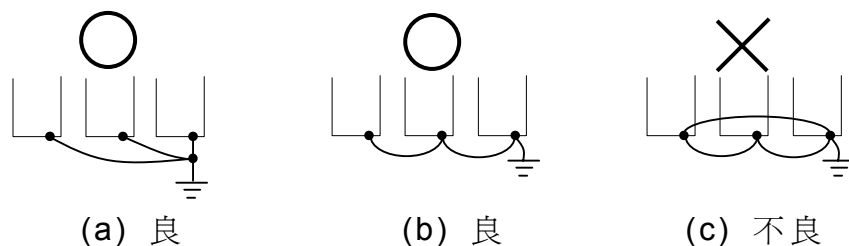
圖 4 7200GS 多台接地方法
